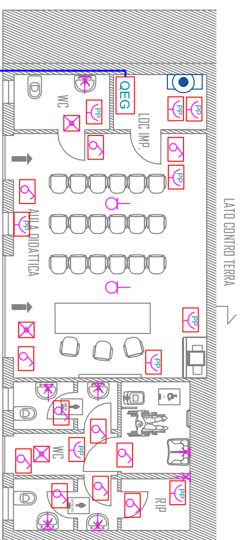
SCHEMA IMPIANTO ELETTRICO _ RAPP. 1:100
